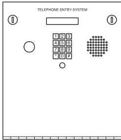
1803 Surface 11.25" W x 13" H x 4.5" D 28.5cm W x 33cm H x 11.43cm D
